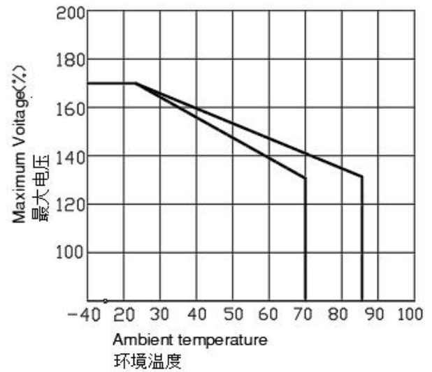
Ambient Temperature vs. Maximum Voltage 环境温度 and 最大电压
