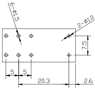
安装图
